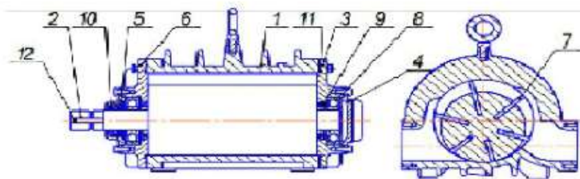
1. Корпус; 2. Ротор; 3. Кришка; 4. Кришка; 5. Кришка; 6. Кришка; 7. Лопатка; 8. Підшипник; 9. Манжета; 10. Манжета; 11. Ущільнююче гумове кільце; 12. Шпонка.
