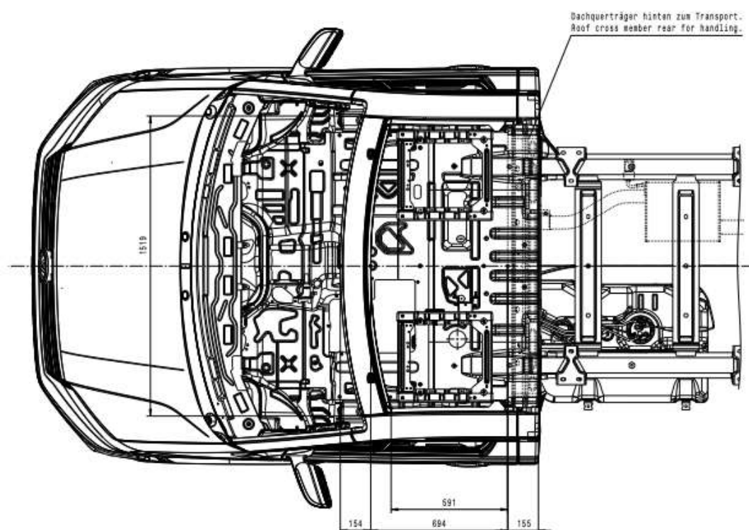
Windlauf ohne Rückwand, ohne Dach Cowl panel without back, without roof
