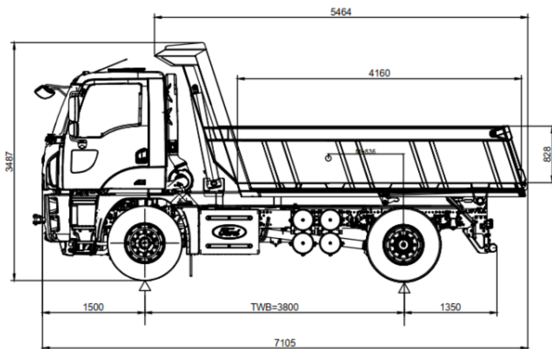
Креслення самоскида на шасі FORD 1833D DC
