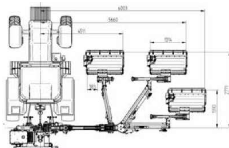
РАДИУС ДЕЙСТВИЯ "ГИДРАВЛИЧЕСКИХ СТРЕЛ" КВТ С ФРЕЗОЙ(СМ)
