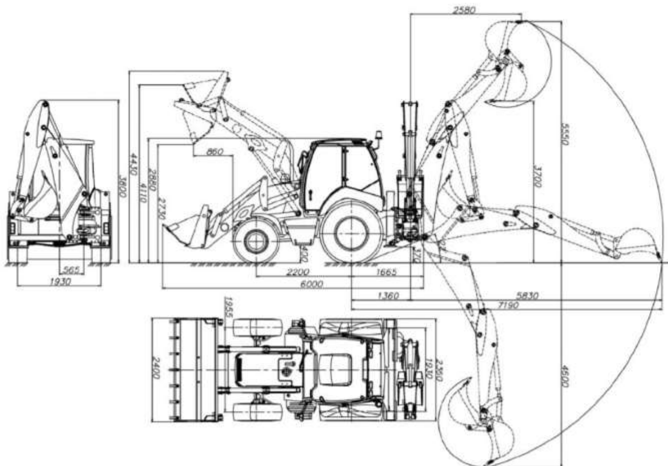
Размерная схема экскаватора – погрузчика Амкодор 732
