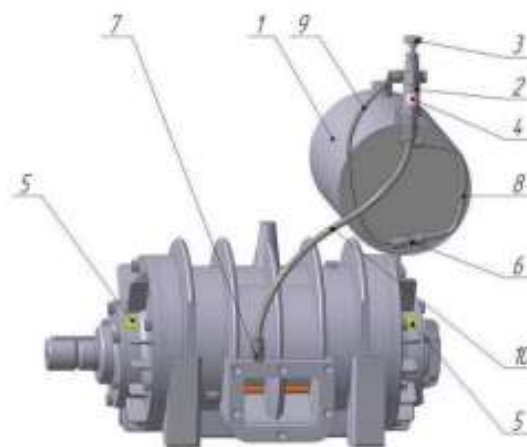
Вакуумный насос
